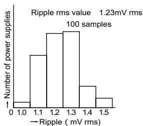
[Fig.-2] Ripple (Noise)
