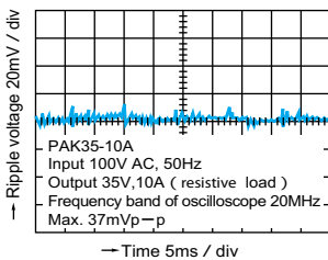
[Fig.-2] Ripple (Noise)
