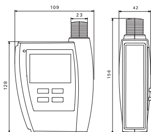
HygroLog HL-NT
